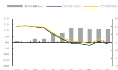
关键期限国债利率（9 月 22 日）
