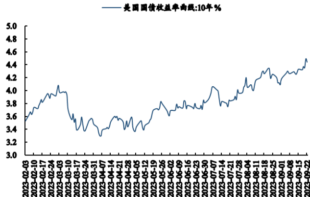
图表32：美债收益率10Y
